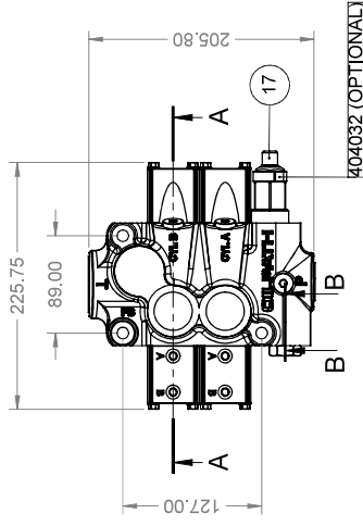
SCALE 1 : 5
